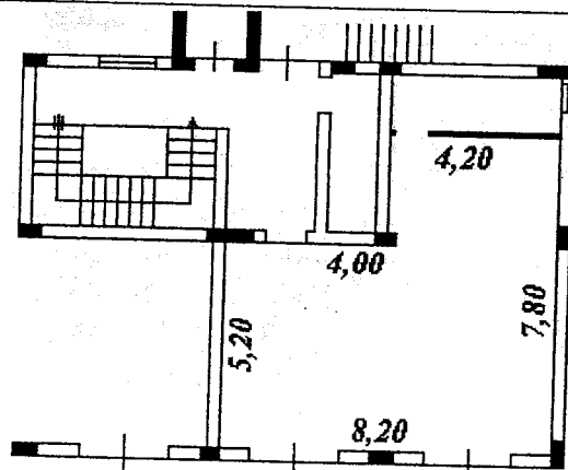
PLANIMETRIA CATASTALE
